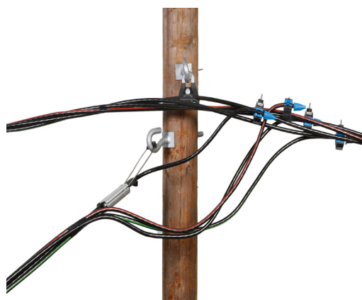
Система СИП-2
